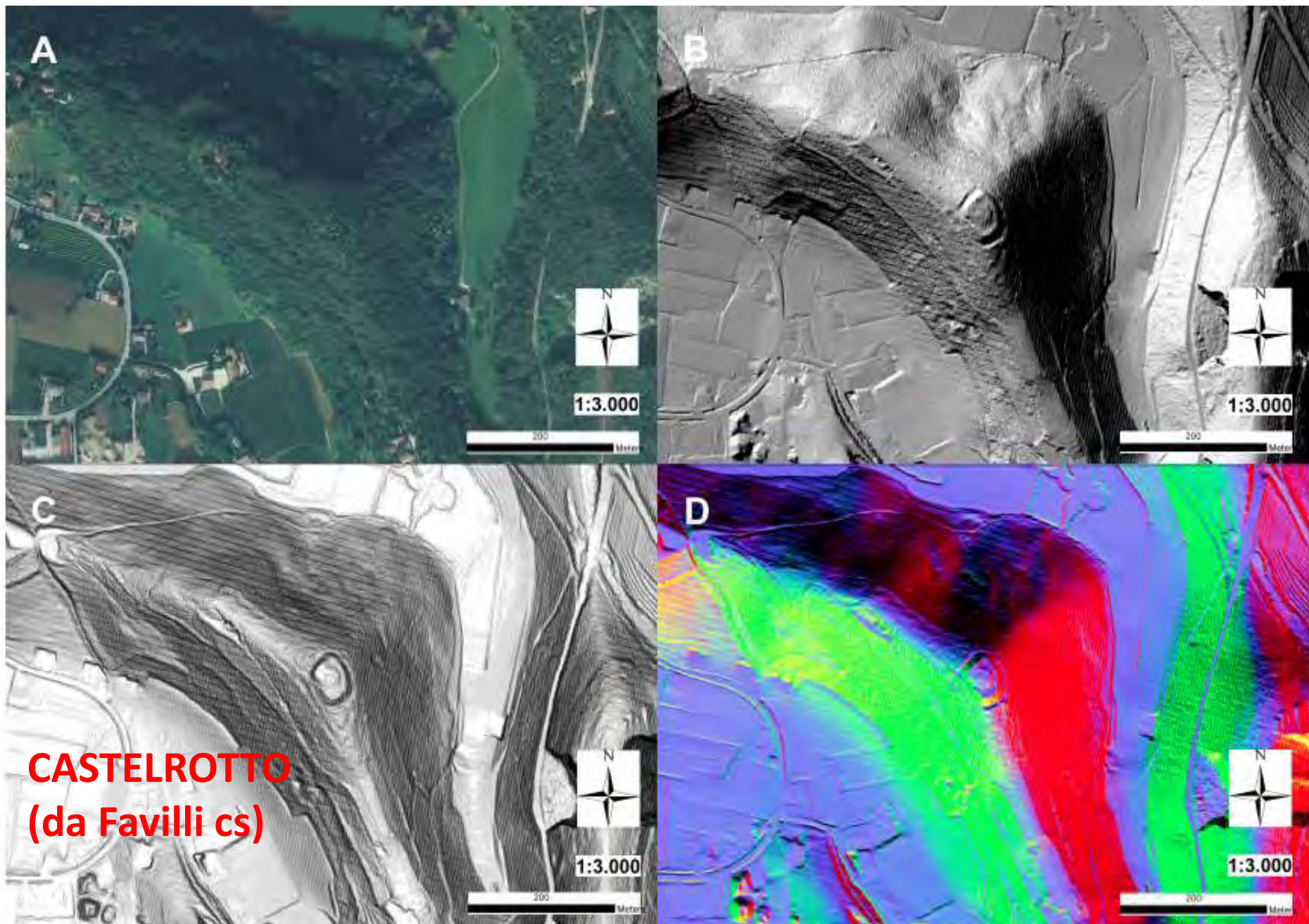
Rovolon, località Castelrotto. (A) Ortofoto a colori 2006, (B) Hillshade, (C) Slopeshade, (D) PCA.
